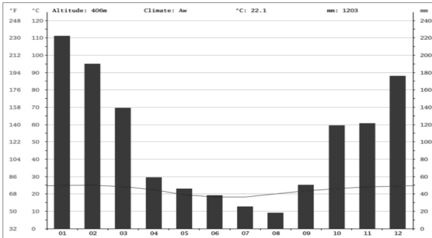
Figura 2 - CLIMOGRAMA DE BIRIGUI
